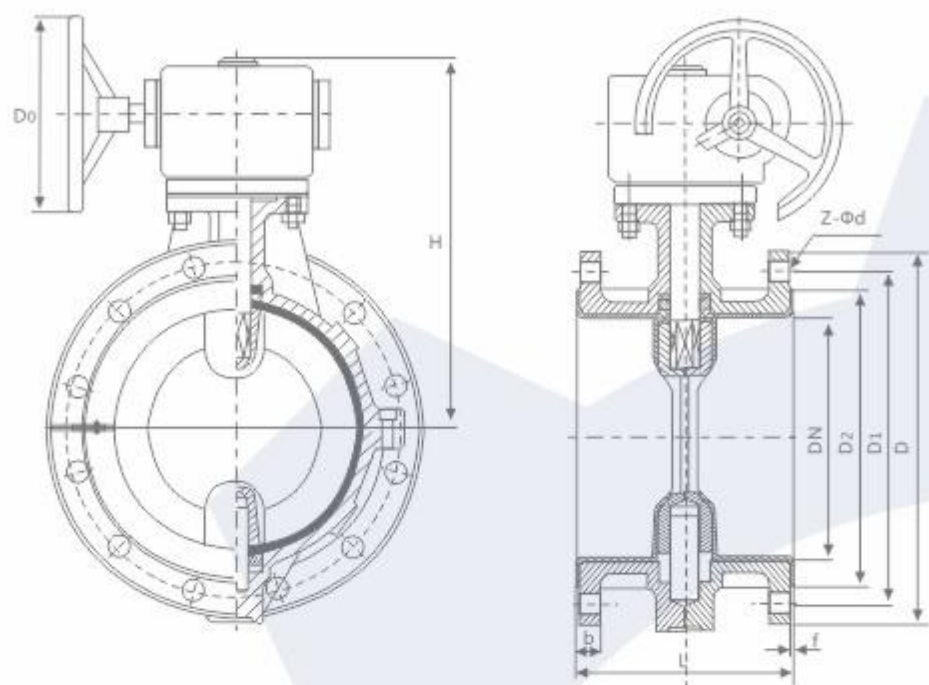
D A 341 F 4 /P 型法兰连接蜗轮传动蝶阀 (中线)
