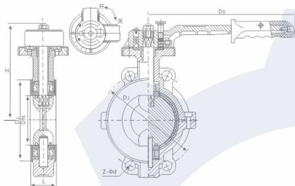
DA71 F4 F46 型对夹式手动蝶阀 (中线)
