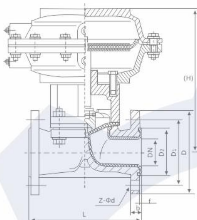
Eg641 F 46 型气动隔膜阀(堰式)
