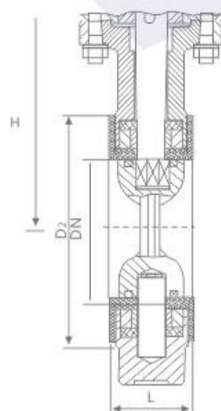
DA371F46型对夹式蜗轮传动蝶阀 (中线)
