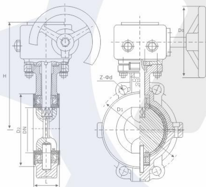
DA371 F4 F46 型对夹式蜗轮传动蝶阀 (中线)
